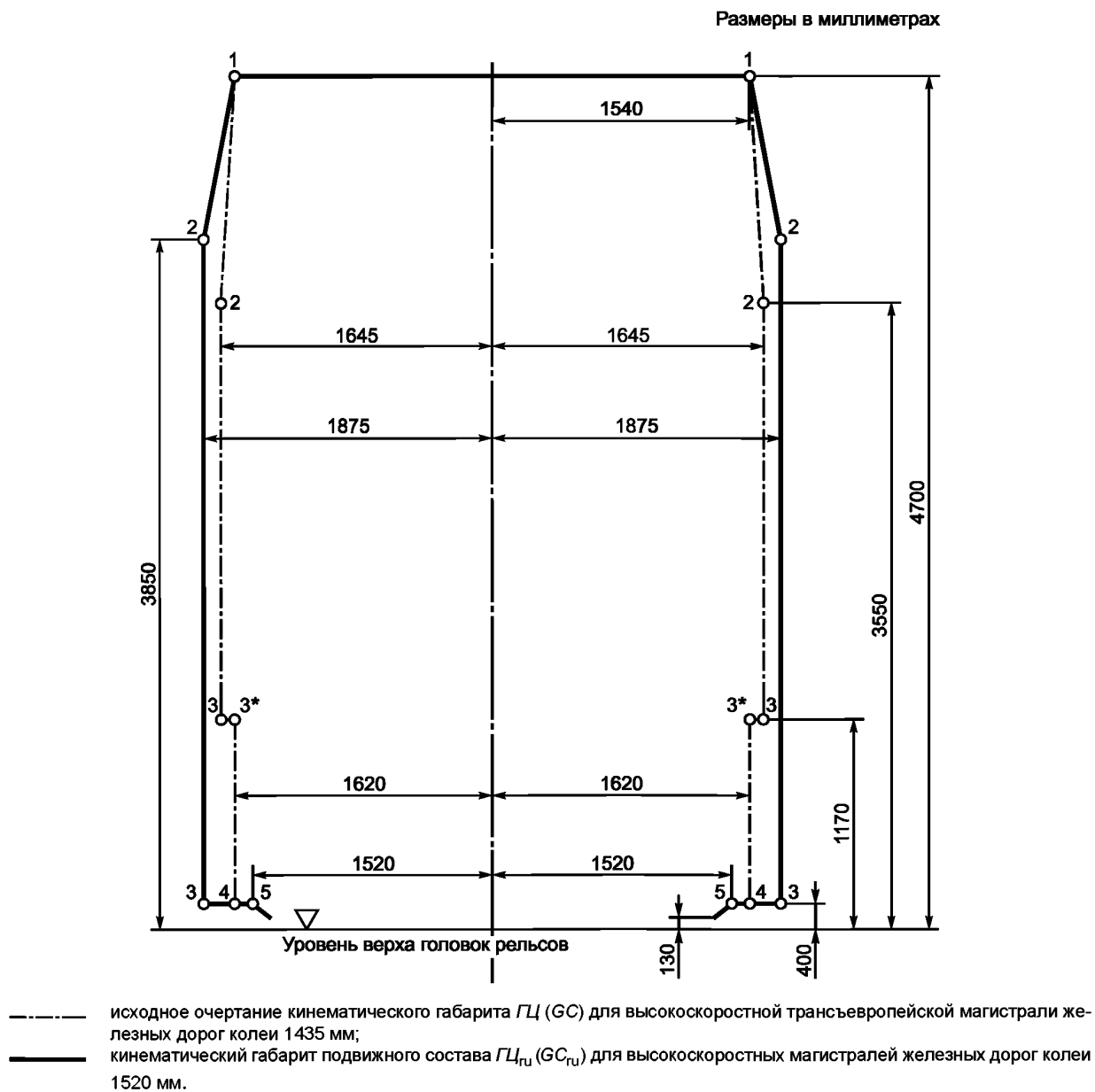
Рисунок 9 — Габарит подвижного состава ГЦ ( GC ) и гармонизированный с ним габарит ГЦ_{ру} ( GC_{ру} )
