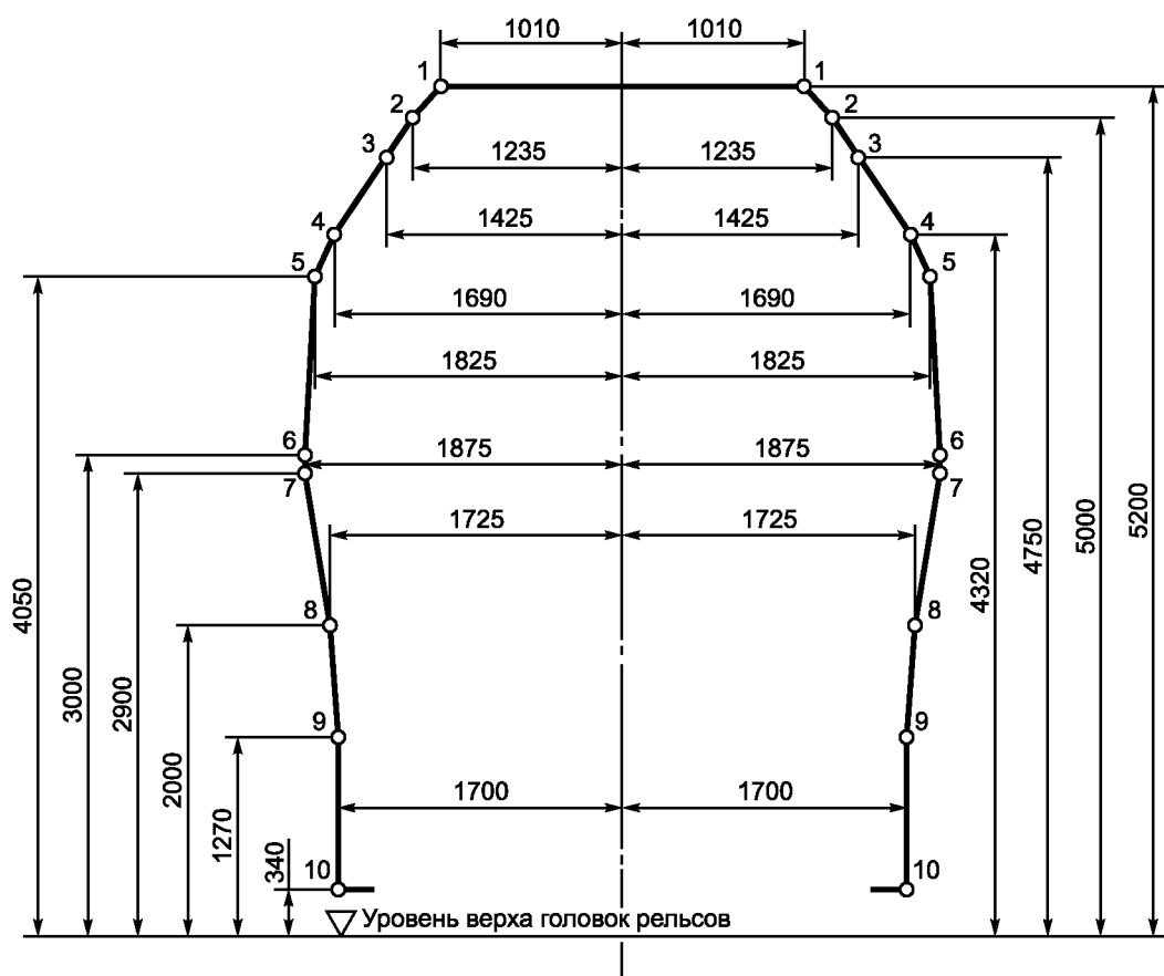
Рисунок 2 — Статический габарит T_{ц}
