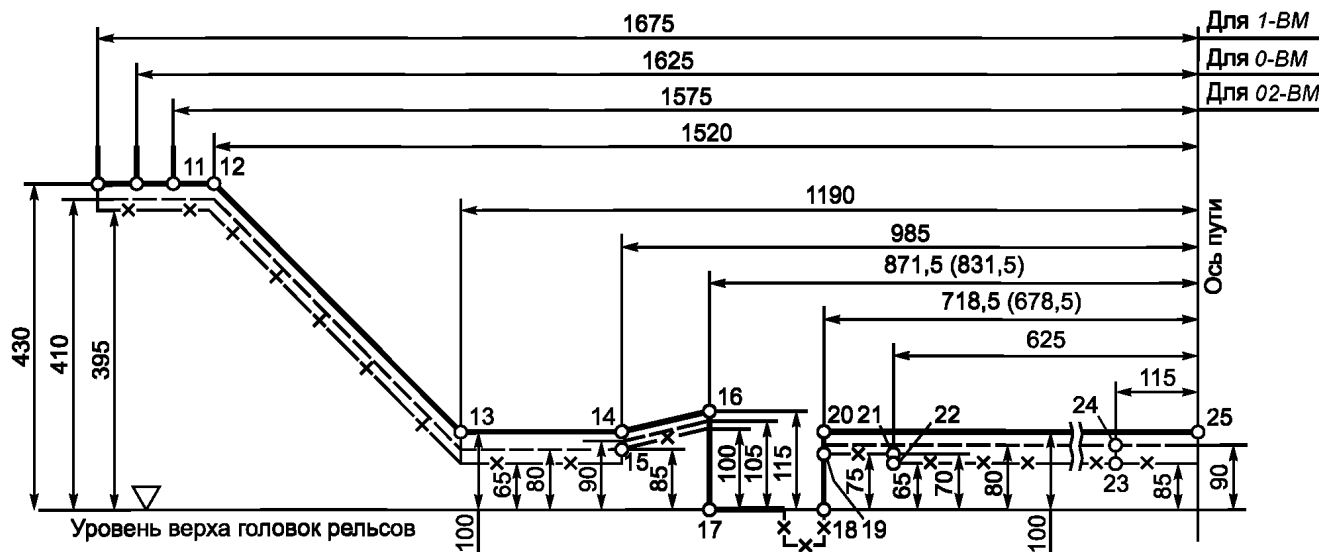
Рисунок 16 — Нижнее очертание габаритов для подвижного состава, проходящего по сортировочным горкам, оборудованным вагонными замедлителями при нерабочем (отторможенном) их положении (включая пути сортировочных горок железных дорог государств-участников СНГ)
