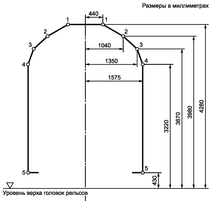
Рисунок 13 — Статический габарит 03-ВМ st
