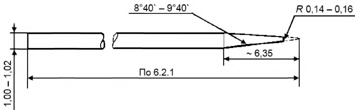
Рисунок 1 – Игла для определения пенетрации
