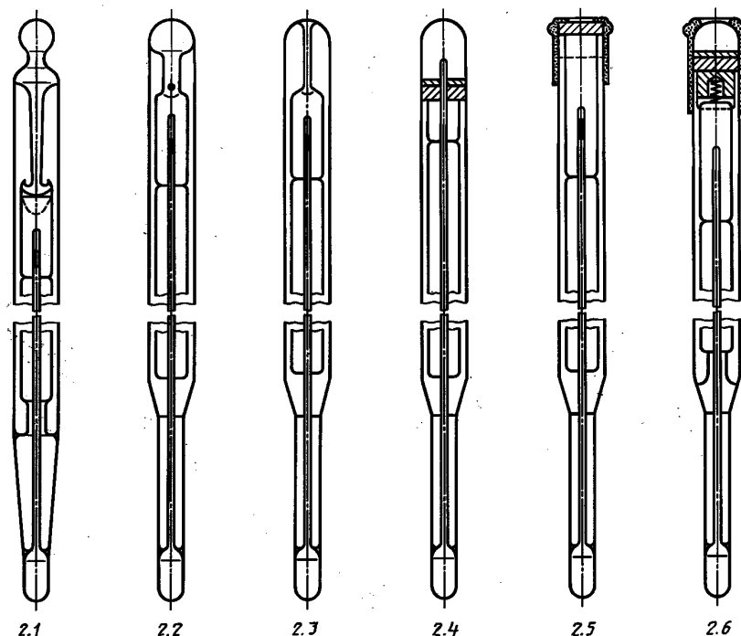
2.1 — со стеклянным седлом и пружиной (по Фуссу); 2.2 — с впаянной стеклянной трубкой (по Рихтеру); 2.3 — с впаянной шпилькой; 2.4 — с пробкой; 2.5 — с пробкой и металлическим копчаком; 2.6 — со стеклянным седлом, пружиной в металлической втулке и копчаком
