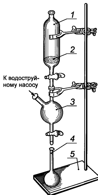
1 — фильтрующая делительная воронка; 2 — втянутый стеклянный фильтр класса ПОР 100 или ПОР 160; 3 — приемник; 4 — мерная колба; 5 — штатив
