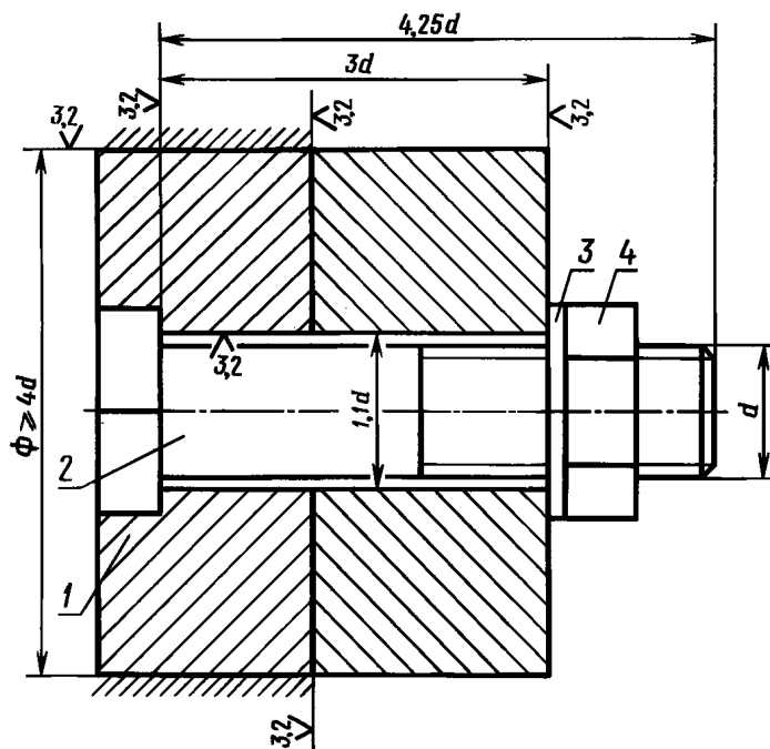
1 — втулка; 2 — болт; 3 — шайба; 4 — гайка
